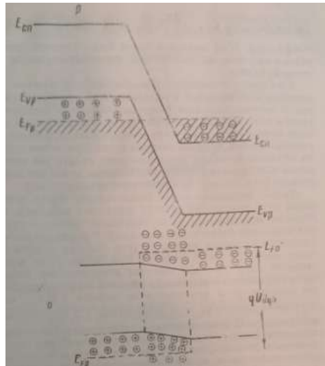
Şəkil 1. Mənfi temperatur halının yaranması a- p-n keçid tarazlıqda ;b-yüksək düzünə gərginlikdə
